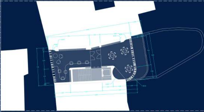
planta primera _Sala subbiblioteca + Lectura infantil
